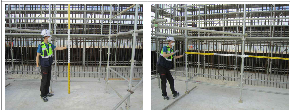
교량 A2 시스템동바리 수직재 및 수평재 간격측정 현황
